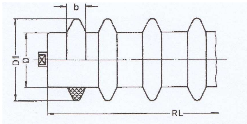
Stützringe pro Rolle
